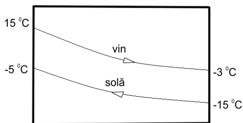
Figura nr. 1.2.1. Circulația fluidelor în schimbătorul de la aplicația 1.1
